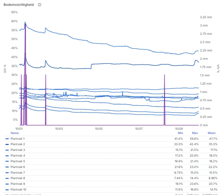
Imaginea 6: Zece senzori de umiditate a solului în diferite tipuri de sol în comparație cu precipitațiile
